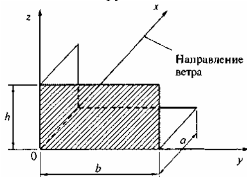
Рисунок 11.2 - Основная система координат при определении корреляции v
