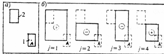
рис.2. Схема к определению дополнительных вертикальных напряжений \sigma_{zp,\alpha} в основании рассчитываемого фундамента с учетом влияния соседнего фундамента методом угловых точек
